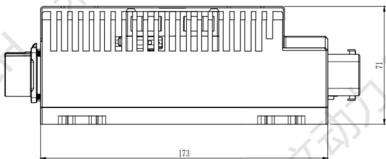
安装孔位图 Mounting Hole(Unit:mm)
