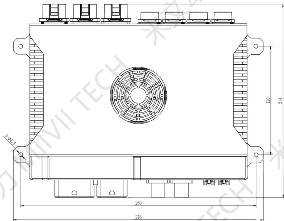
主视图 Front view(Unit:mm)
