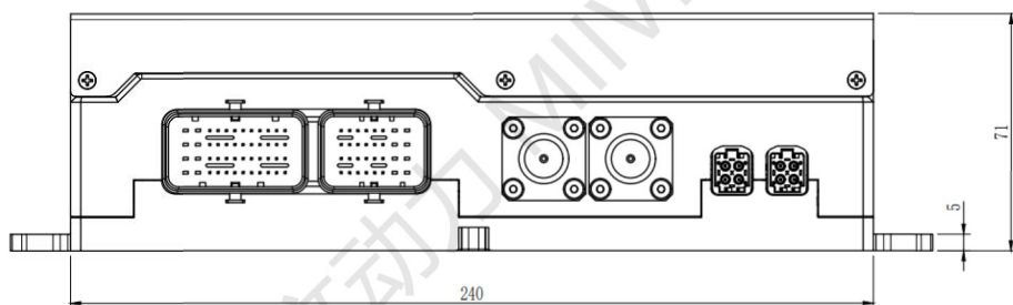
左视图 Left view(Unit:mm)
